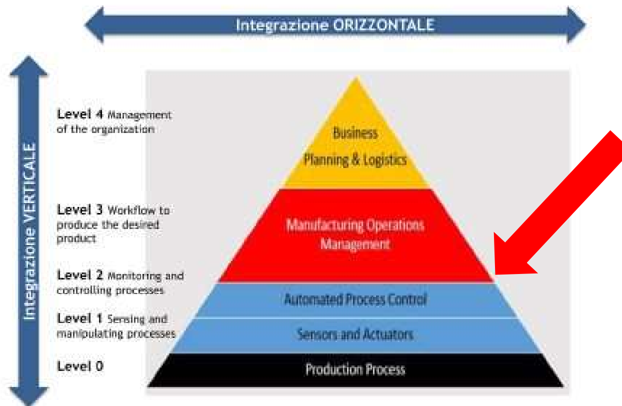
Architettura a livelli ISA 95 (IEC 62264)
